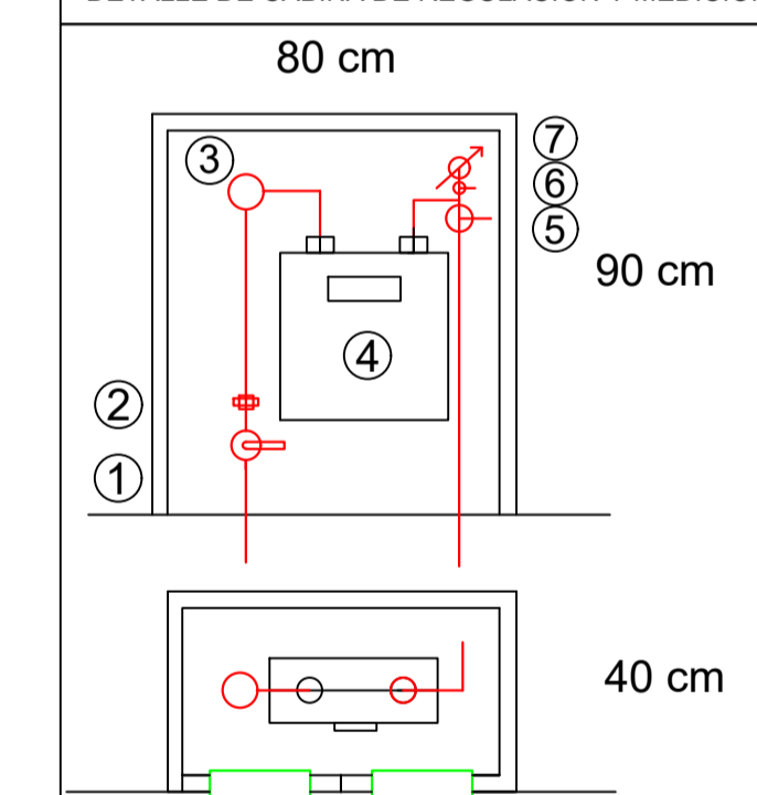
DETALLE DE CABINA DE REGULACIÓN Y MEDICIÓN
