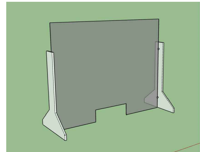
LATERALES MELAMINA BLANCA SOBRE MDF 12 MM
