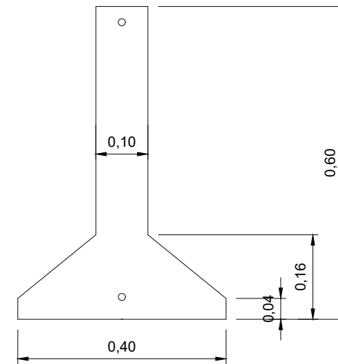
LATERALES MELAMINA BLANCA SOBRE MDF 12 MM
