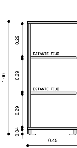
CORTE A-A
