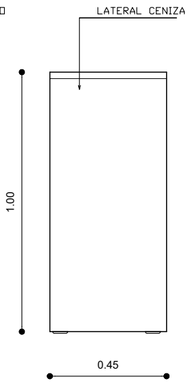
VISTA LATERAL
