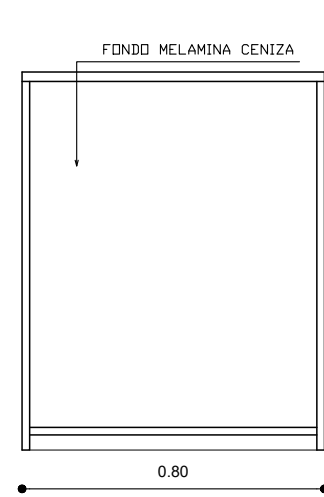
VISTA POSTERIOR
