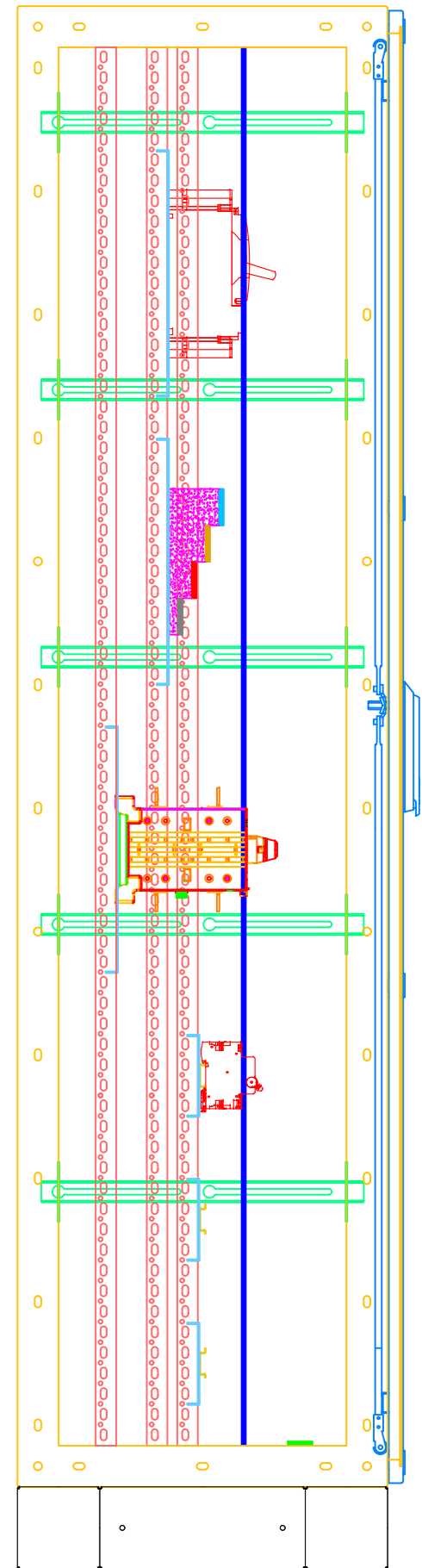
VISTA LATERAL MÓDULO N°7
