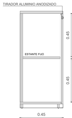
CORTE A-A
