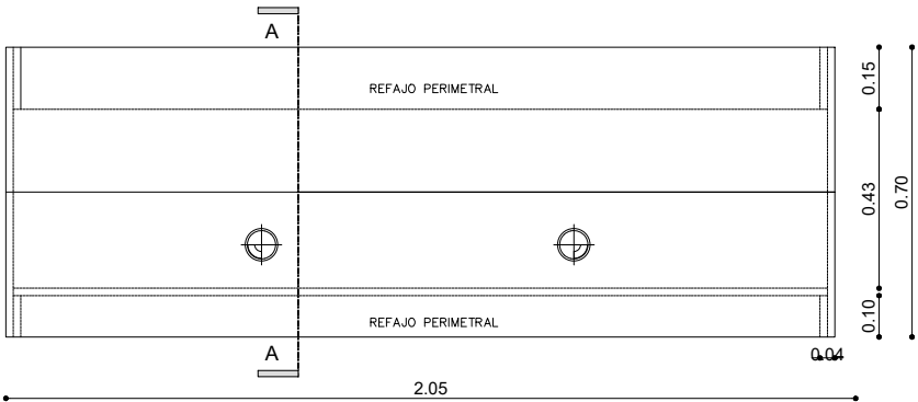
VISTA SUPERIOR
