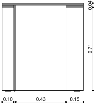
CORTE A-A
