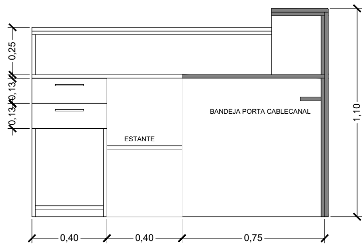
CORTE A-A
