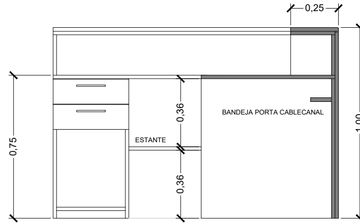
CORTE B-B
