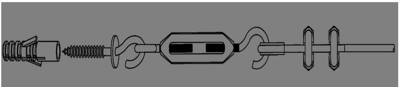
DETALLE CON TENSOR
