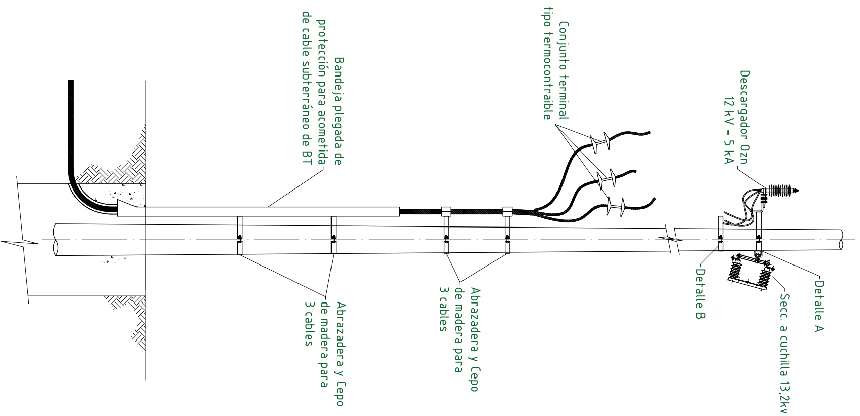
Acometida de cable subterráneo TN120 Esc. 1: 40
